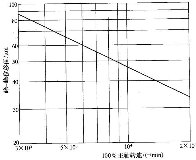
图 1 允许最大轴振动的数量值指导性线图
